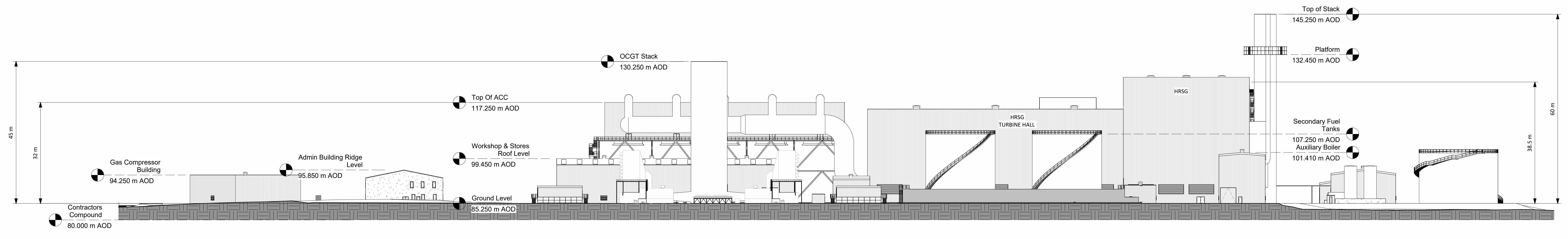
4 South 1 : 500
